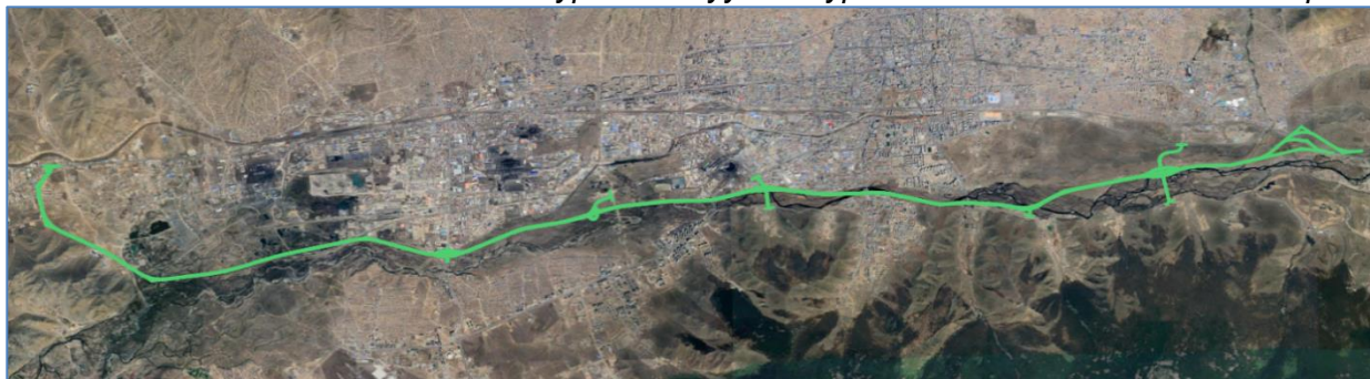
Зураг 26. Туулын хурдны замын төлөвлөлтийн трасс.
