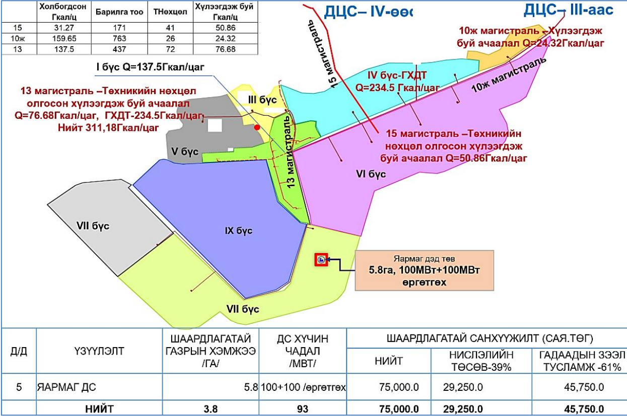
Зураг 16. Нисэх, Яармагийн ХЕТ-ний дулаан хангамжийн төлөвлөлт.
