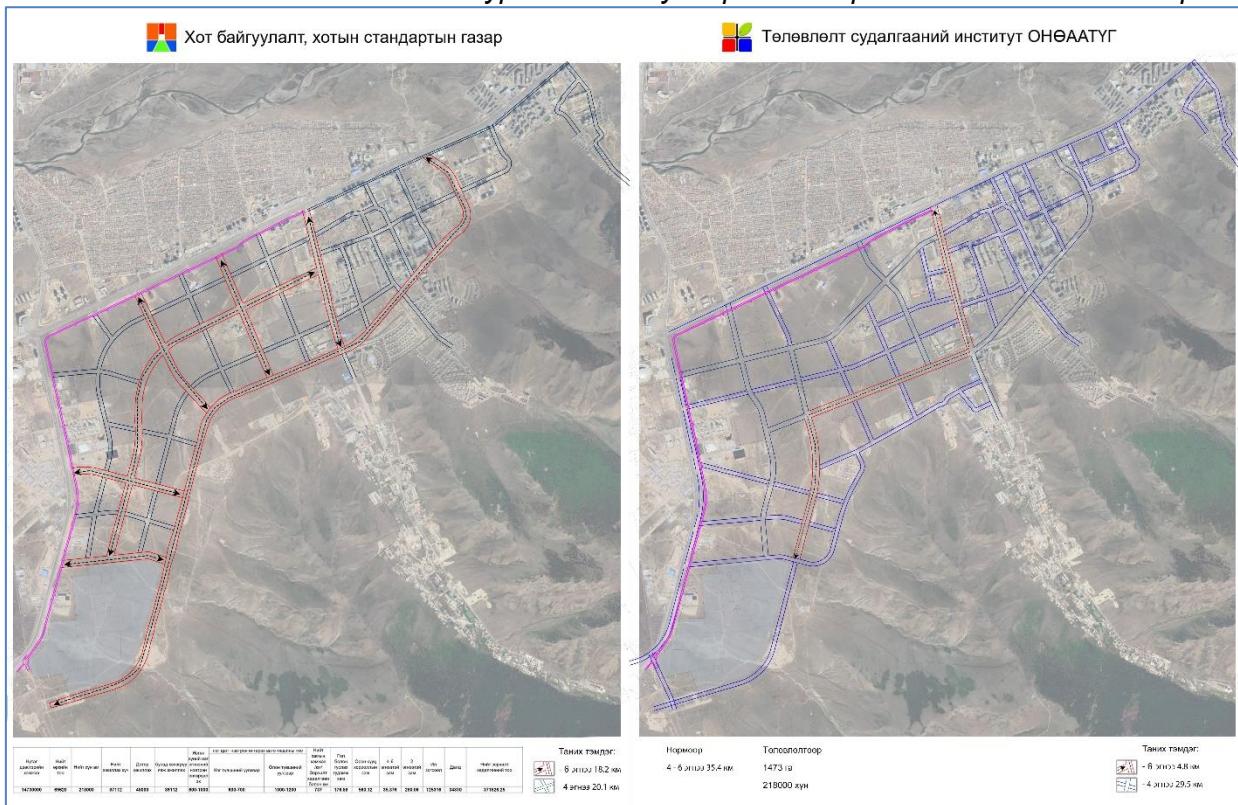
Зураг 49. 27 дугаар нэгж хорооллын авто замын трасс.
