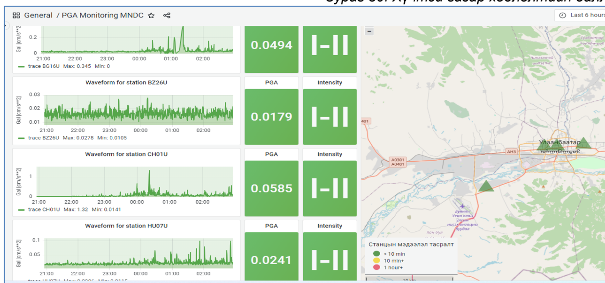
Зураг 30. Хүчтэй газар хөдлөлтийн балл.
